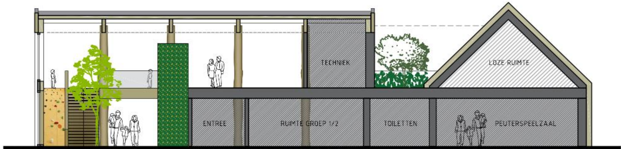
Principe - langsdoorsnede
